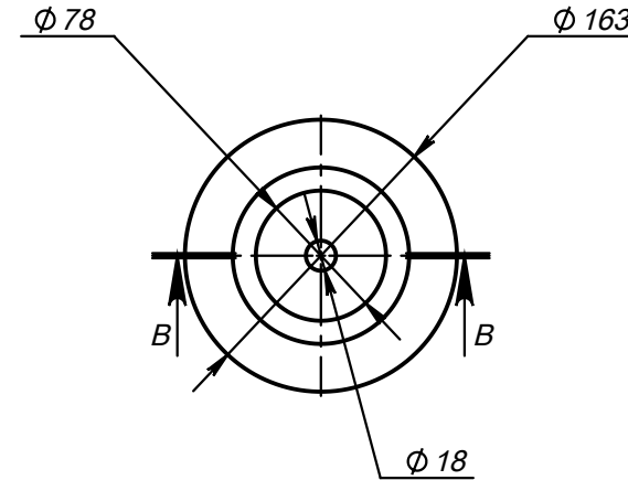
Поз.3 (Тарелка)
