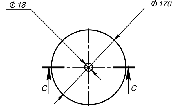
Поз.2 (Основание нижнее)
