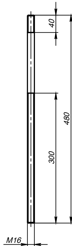
Поз.4 (Шпилька)
